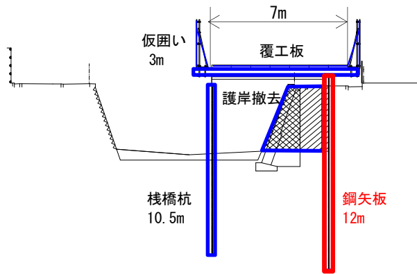
栈橋断面図
