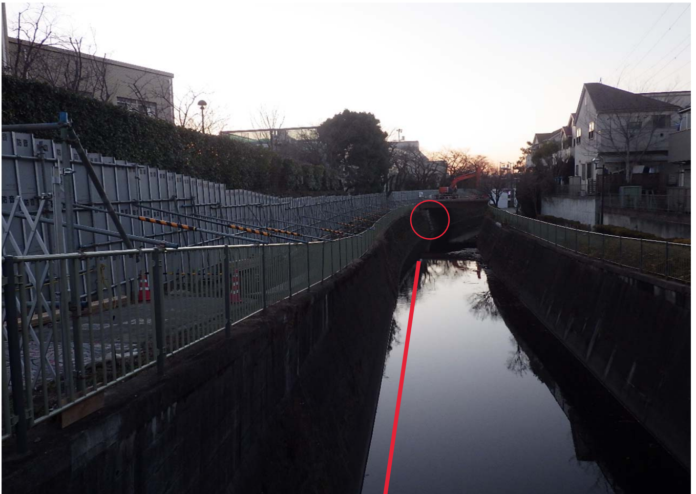
下流側(永福橋より望む)：護岸撤去工
