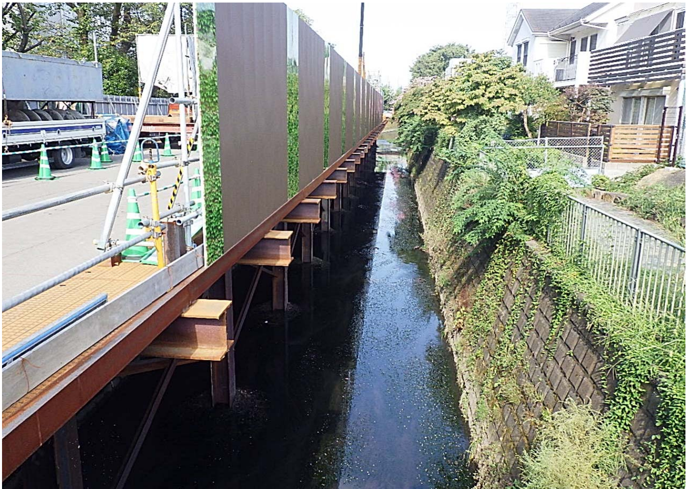
かな橋側：栈橋設置・護岸撤去工 103m完了
