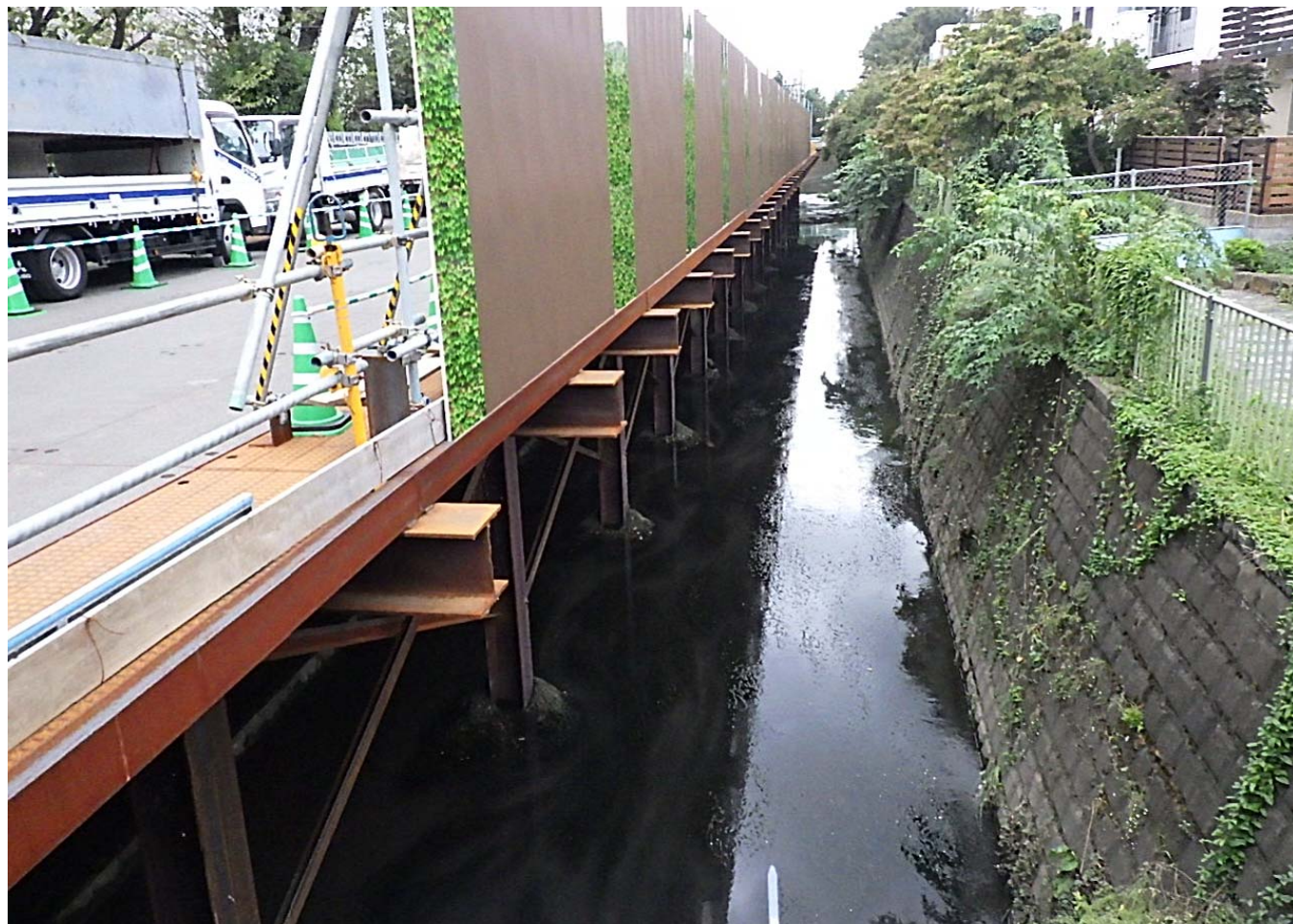
かな橋側：栈橋設置・護岸撤去工 109m完了
